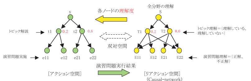
図2 Causal-networkを利用したユーザ適応化の原理
