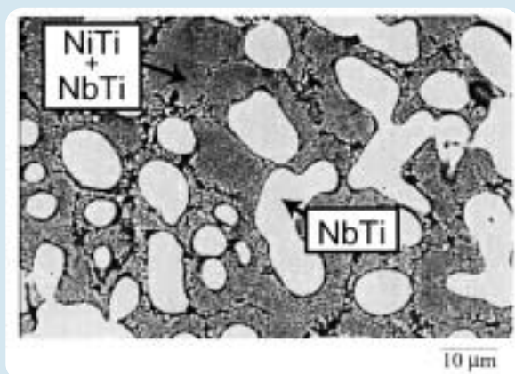
図2 Ni 30 Ti 31 Nb 39 合金のSEM写真。白い部分は初晶のbcc-NbTi相。層状の微細組織はNiTi-NbTiの共晶。
