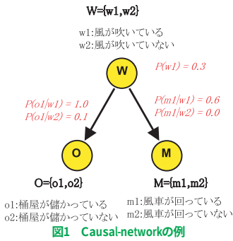
図1 Causal-networkの例
